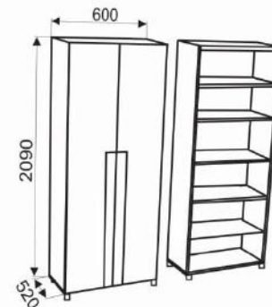
Dulap 0,6m
