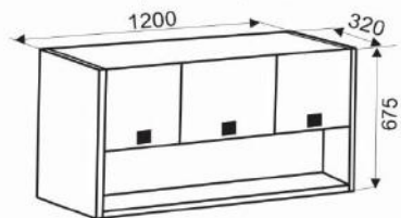
Suspendat 1,2m
