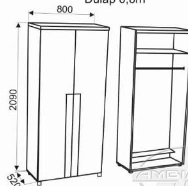
Dulap 0,8m
