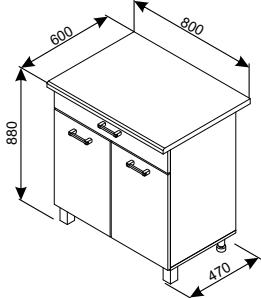
800 BI Modul inferior (sertar + usi)
