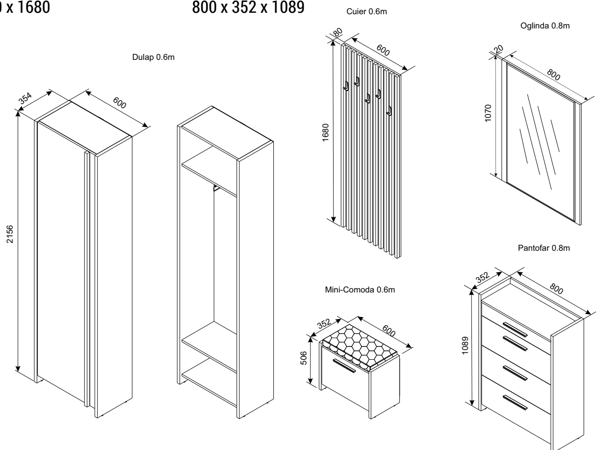
Cuier / Hanger: 600 x 80 x 1680
