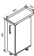
MI 7 Modul inferior 200
