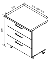
MI 1 Modul inferior 400/600/800
