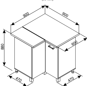
CI Modul inferior (de colț)
