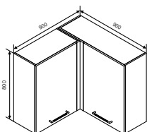
MS 8 Modul superior 900
