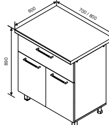
MI 9 Modul inferior 700/800
