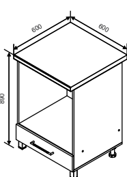
MI 2 Modul inferior 600
