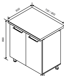
MI 5 Modul inferior 700/800
