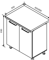
MI 4 Modul inferior 600/800
