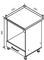
MI 2 Modul inferior 600
