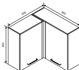
MS 8 Modul superior 900
