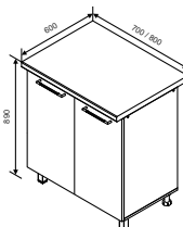
MI 5 Modul inferior 700/800
