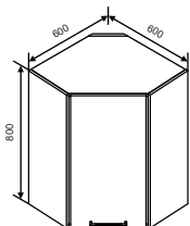
MS 8 Modul superior 600
