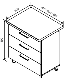
MI 1 Modul inferior 400/600/800
